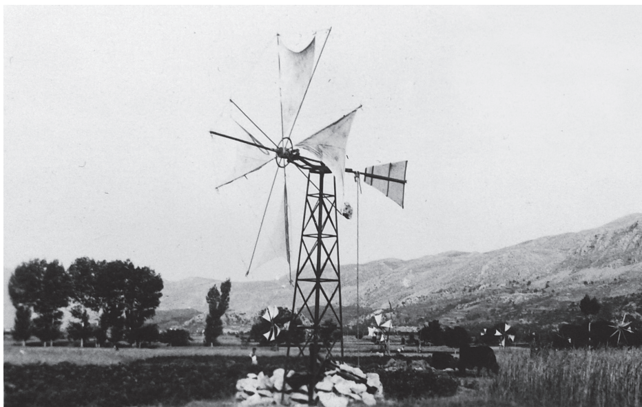
Μεταλλικός ανεμόμυλος ποτίσματος στο Οροπέδιο. Φωτογραφία δεκαετίας 1930.
