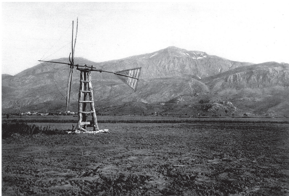
Ξύλινος ανεμόμυλος του Οροπεδίου Λασιθίου. Εφεύρεση του Εμμανουήλ Παπαδάκη περί το 1890. Τεχνικές βελτιώσεις του ανεμόμυλου έγιναν μετά το θάνατό του από το μαθητή του Στέφανο Μαρκάκη ή Μαρκοστεφανή και από το γιο του Γεώργιο Παπαδάκη. (Φωτογραφία από το βεύκωμα GRIECHENLAND του Dr. HELMUTH TH. BOSSERT, BERLIN 1928)
