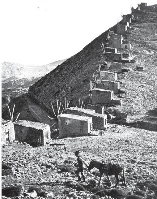
Οι αλευρόμυλοι στη βόρεια είσοδο του Οροπεδίου, από τους οποίους ο Εμμανουήλ Παπαδάκης εμπνεύστηκε τον αντλητικό ανεμόμυλο, το λεγόμενο και ανεμόμυλο ποτίσματος ή ανεμαντλία. (Φωτογραφία της δεκαετίας του 1930)
